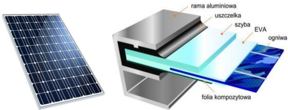
Rysunek 2. Pojedynczy moduł fotowoltaiczny oraz jego przekrój.
