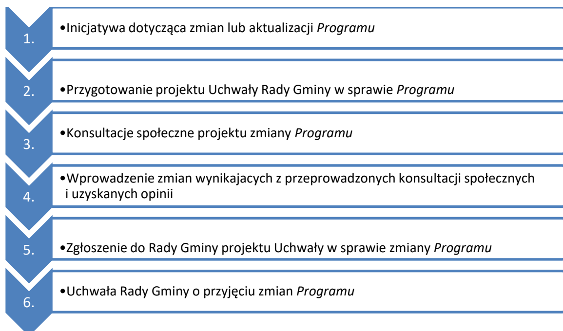
Rys.11.Aktualizacja Programu
